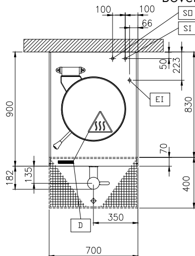
Boven aanzicht
